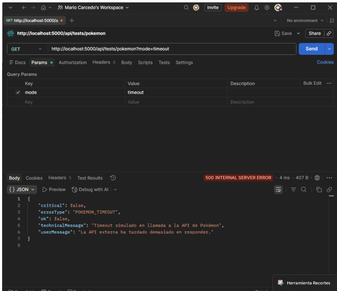
Ilustración 9 - Timeout / error remoto
