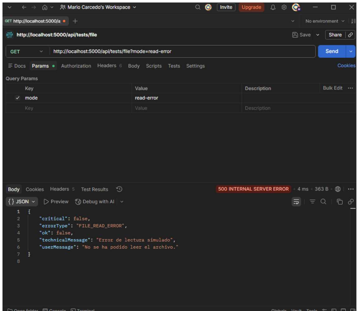
Ilustración 3 - Error de lectura
