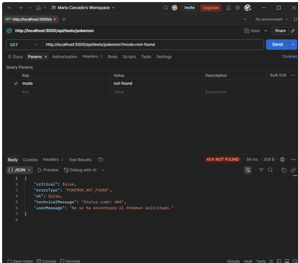
Ilustración 8 - Pokémon no encontrado
