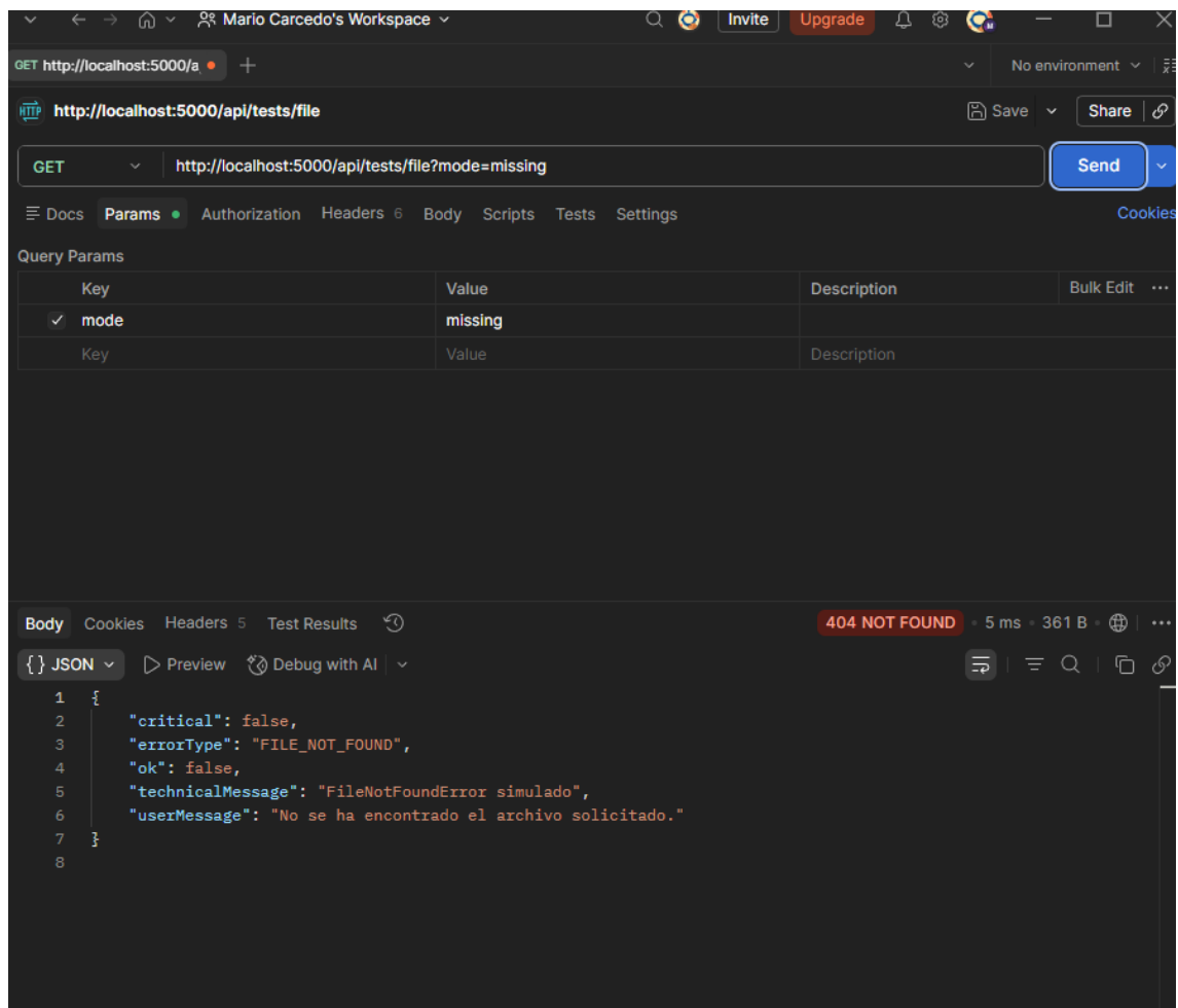
Ilustración 2- Archivo no encontrado
